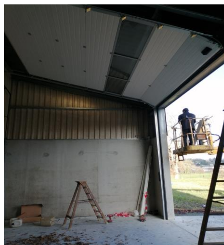
Nouvelle ouverture créée sur la droite du bâtiment Charlieu
