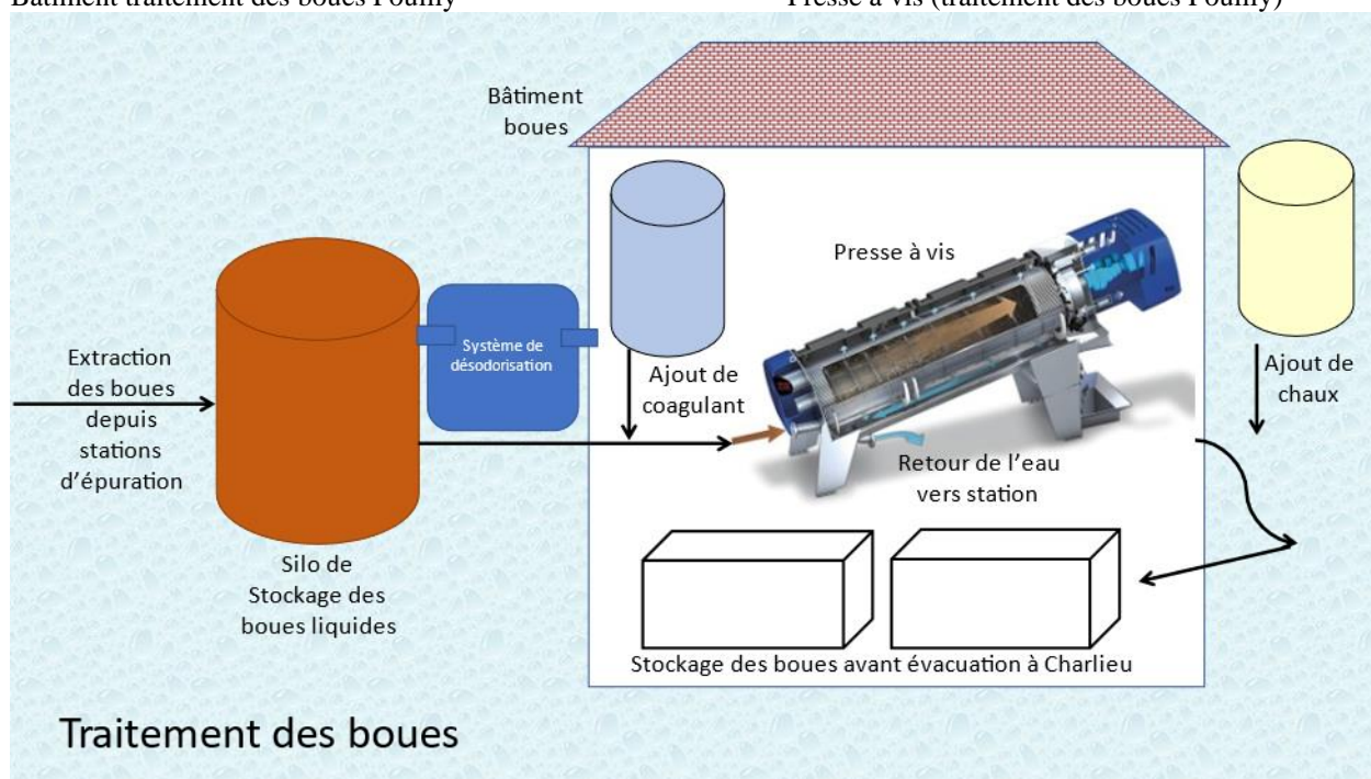
Bâtiment traitement des boues Pouilly
